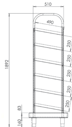
MEDIDAS DISPENSADOR DE PIE
